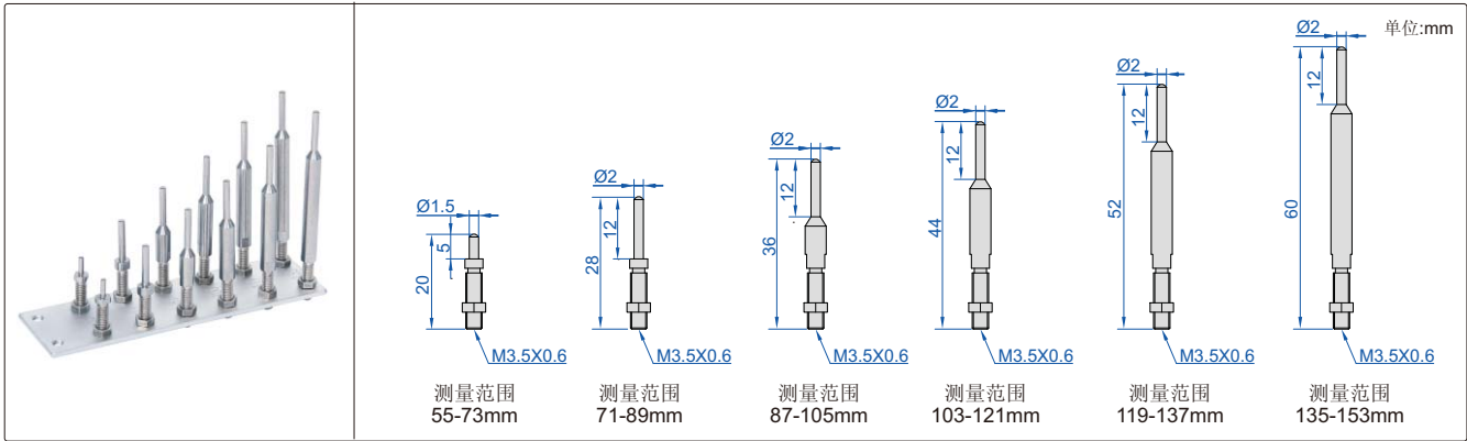
2223-153测头(标配)
