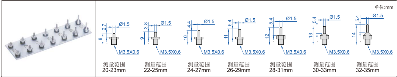
2223-35测头(标配)
