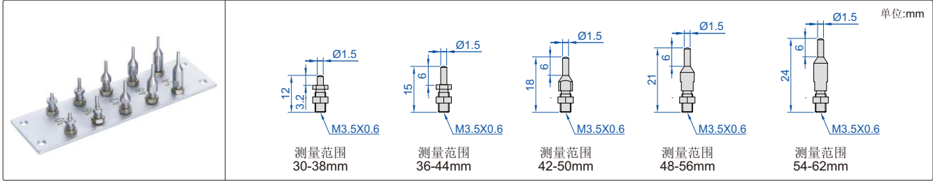
2223-62测头(标配)
